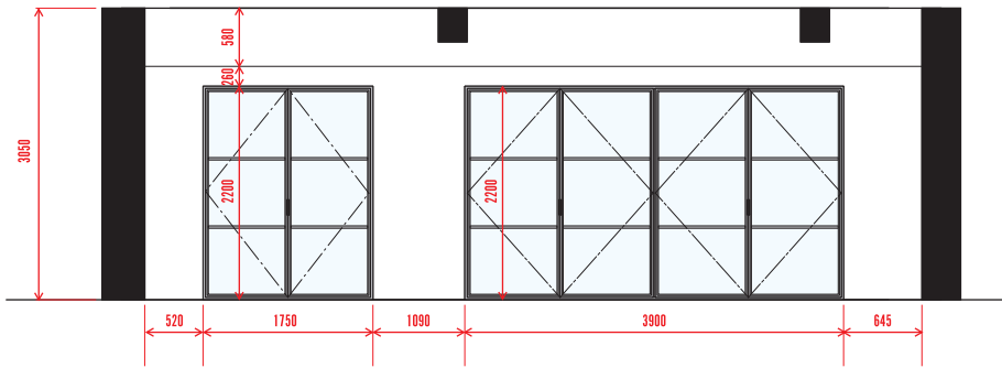
Elevation - A
