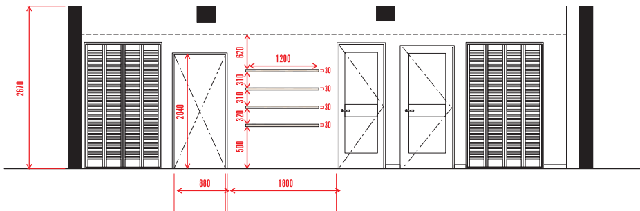
Elevation - C
