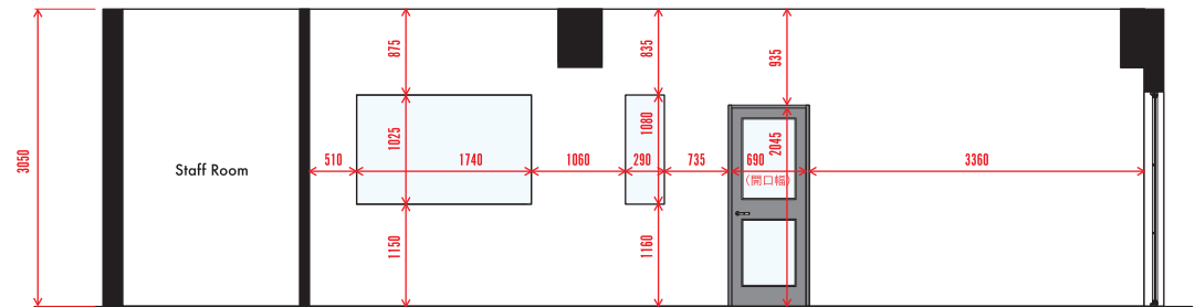
Elevation - D
