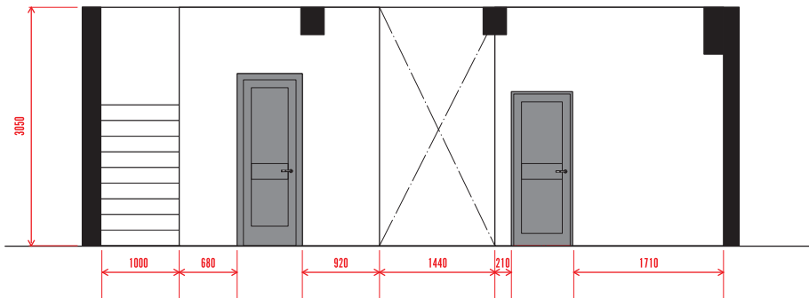
Elevation - C
