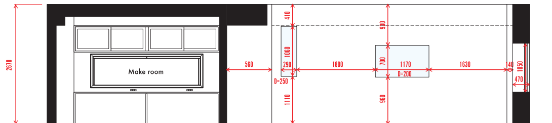
Elevation - D
